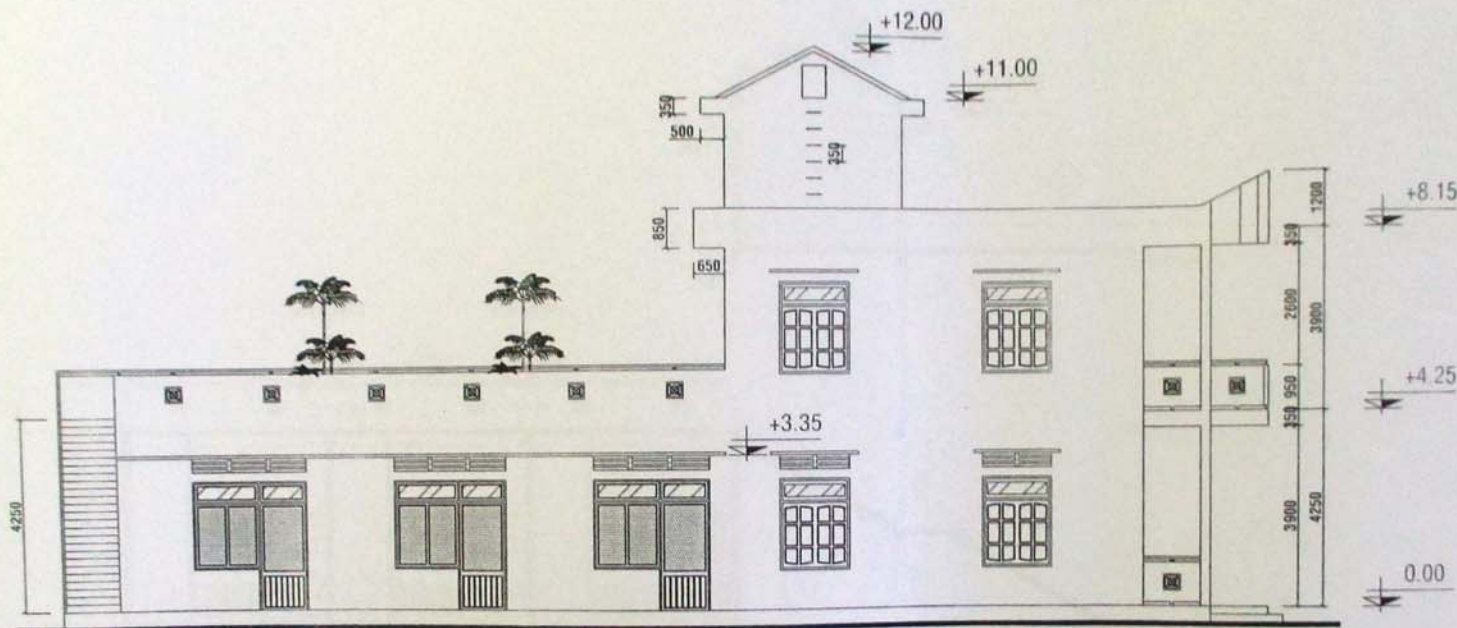
MẶT ĐỨNG TRỤC G-A
