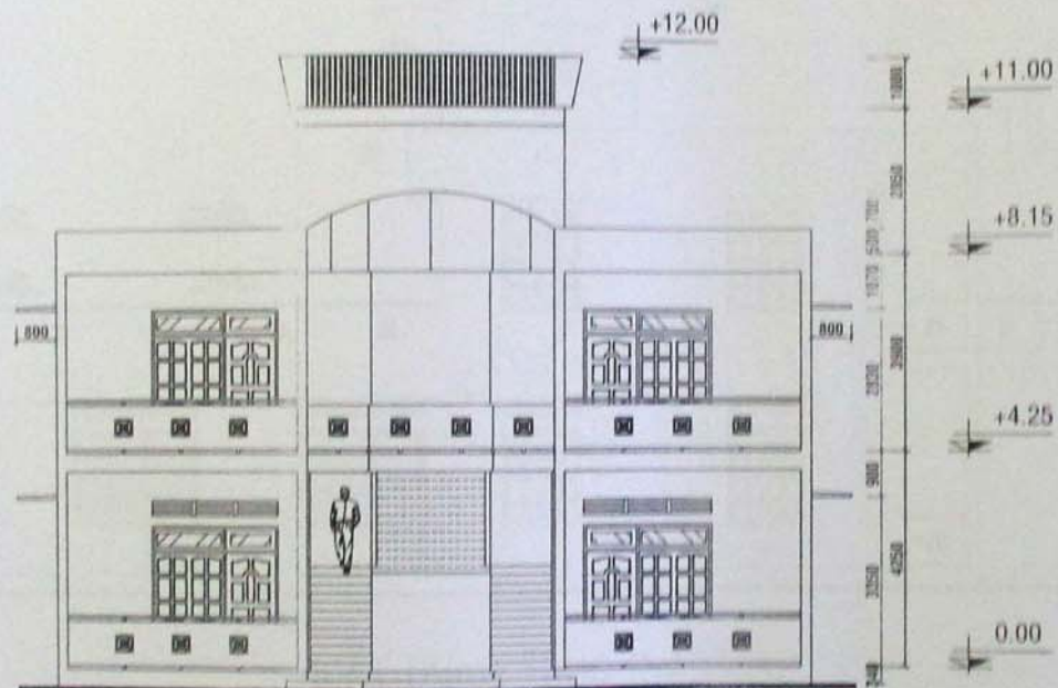
MẶT ĐỨNG TRỤC 1-4
