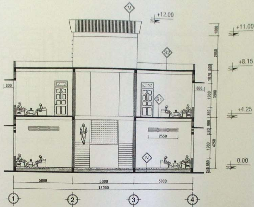
MẶT CẮT B-B
